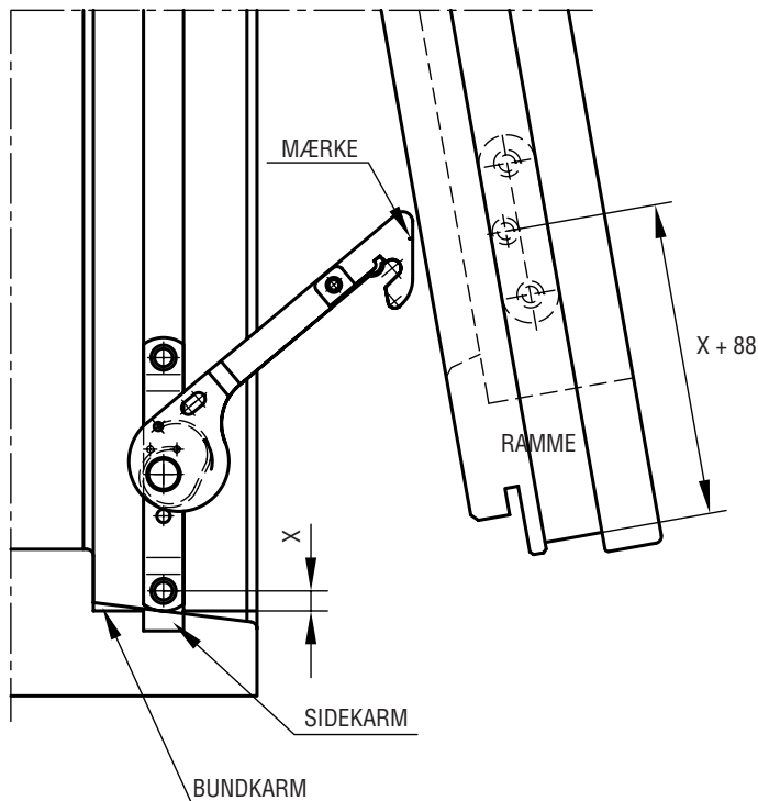
FIG. 1 VIST SOM HØJRE (SET UDEFRA)
